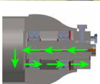
LAUFWALZE
