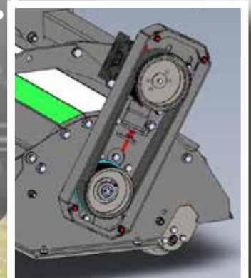
POWERBELT ANTRIEBSRIEMEN
